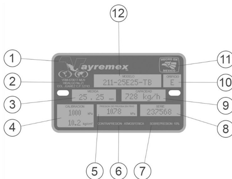
Fig.2 Formato de placa de identificación
