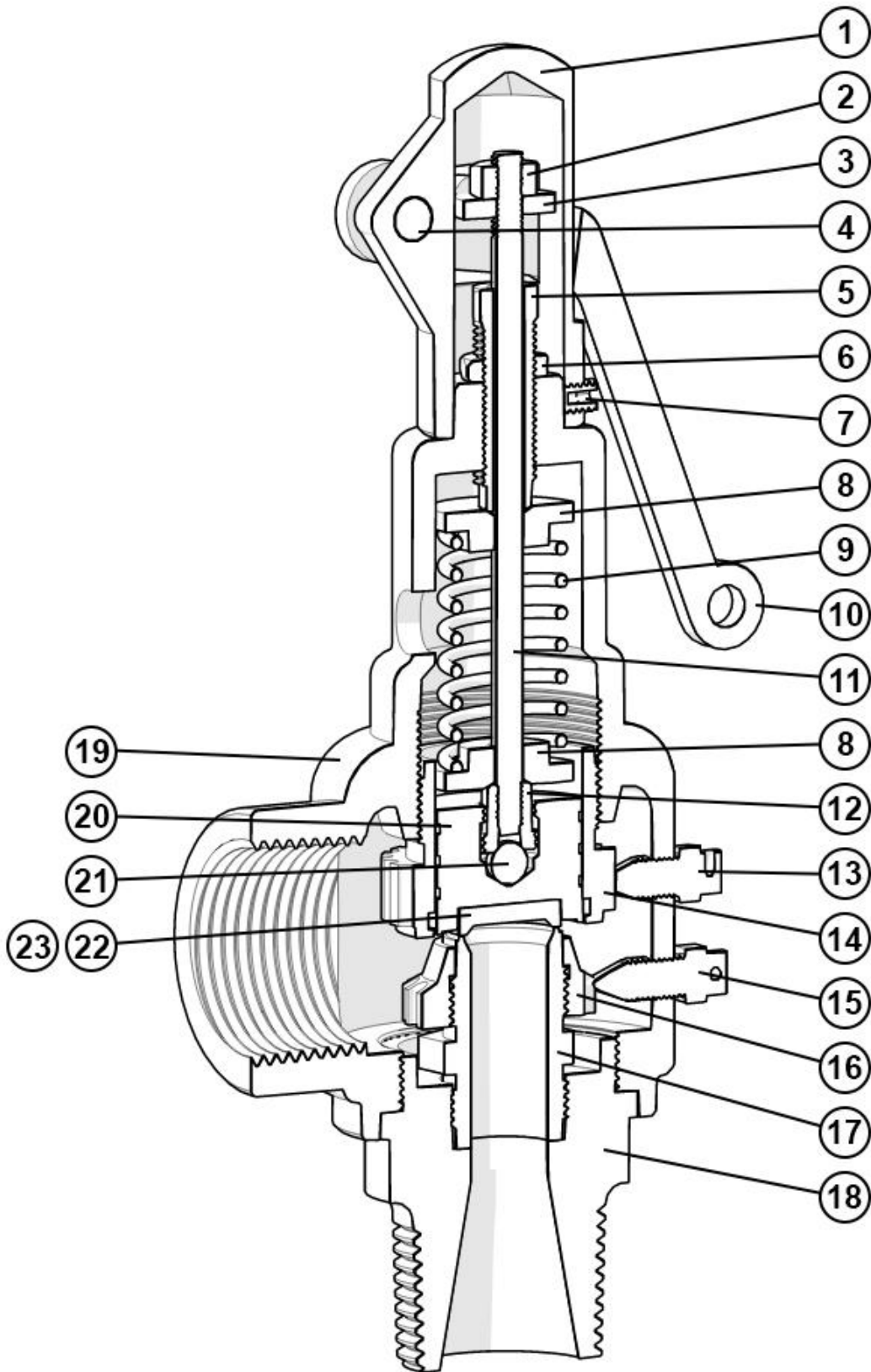
Fig.1 Seccionado de válvula de seguridad modelo 211 estándar
