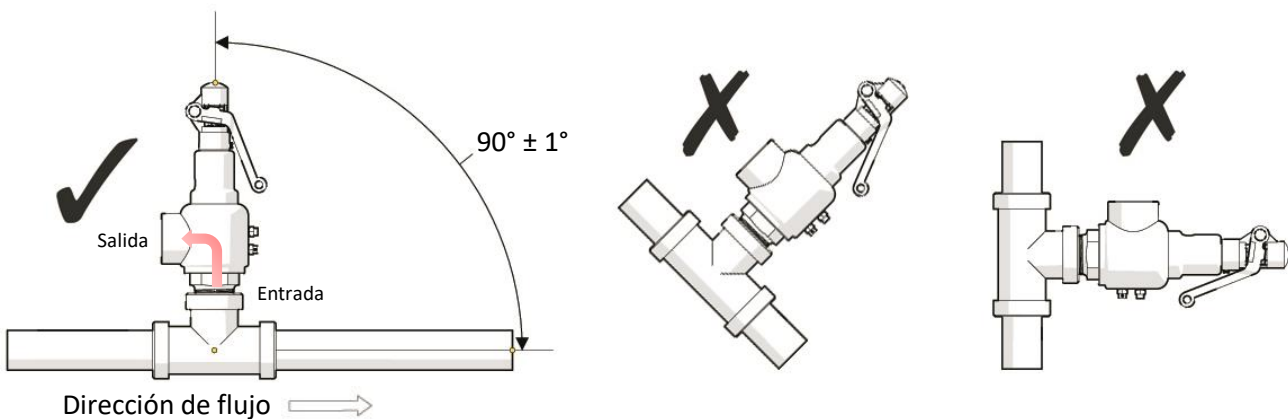
Fig. 3 Posición y orientación correcta de una VRP
