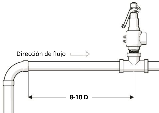
Fig. 5 Distancia recomendada entre la válvula y cualquier dispositivo
