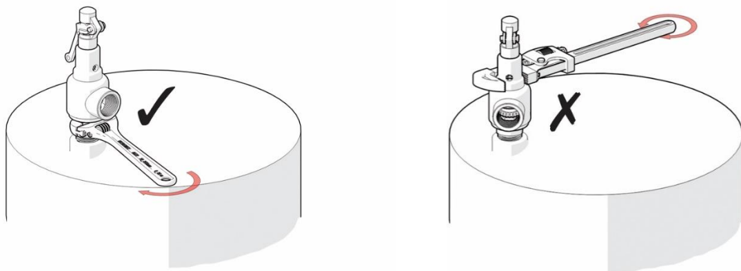
Fig. 6 Forma correcta de conectar/desconectar la válvula de seguridad
