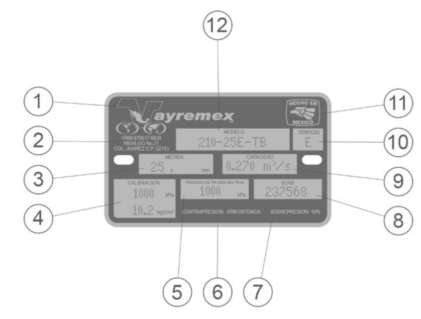
Fig.2 Formato de placa de identificación
